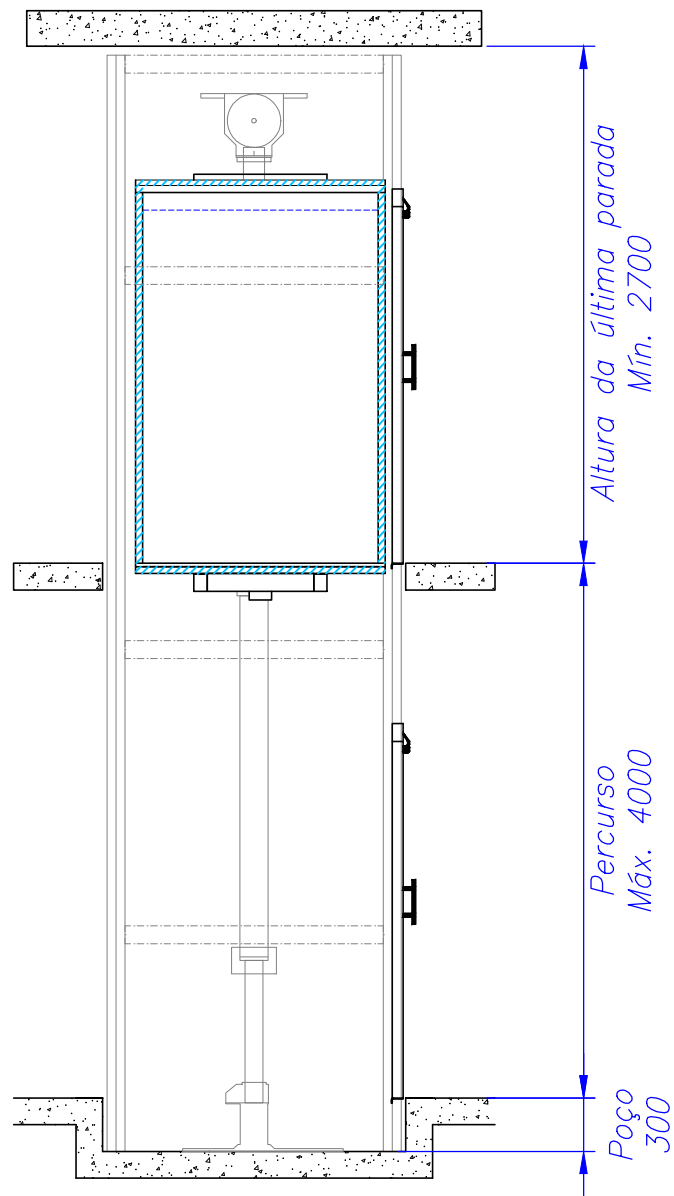
CORTE ESQUEMÁTICO
