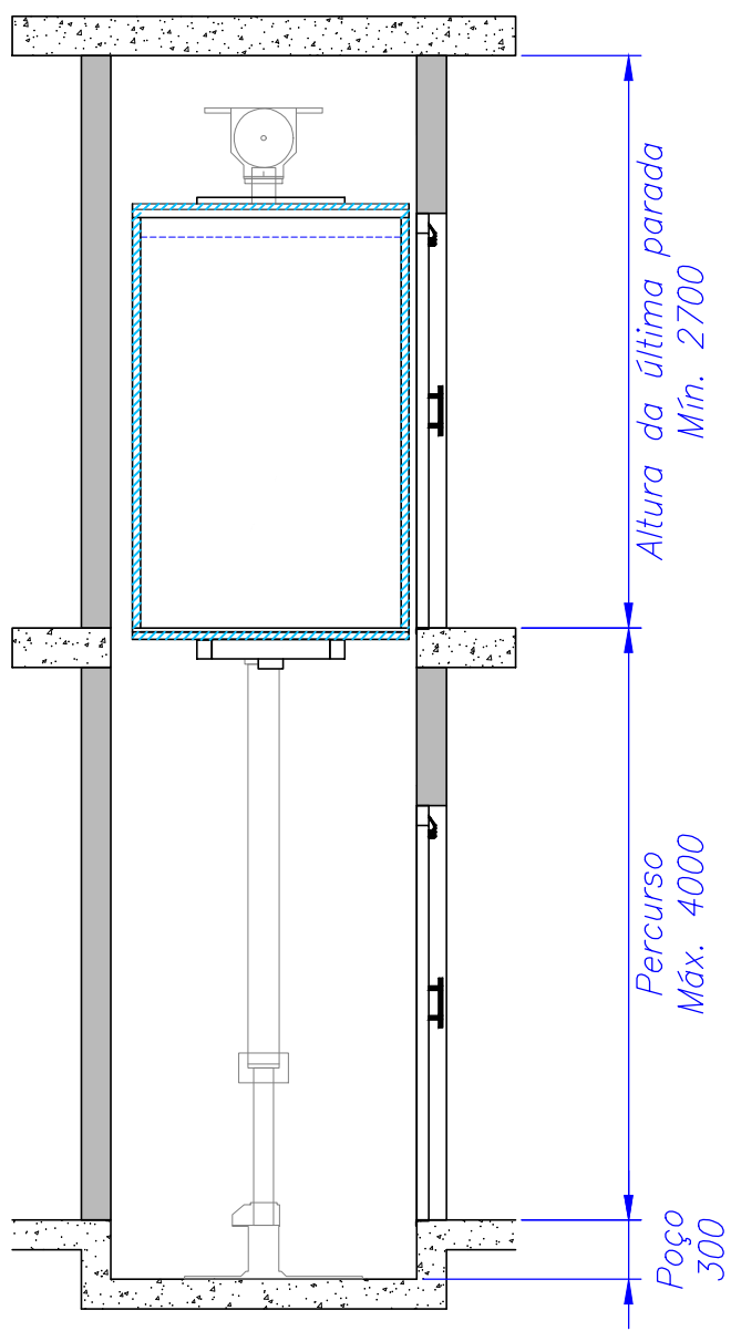
CORTE ESQUEMÁTICO
